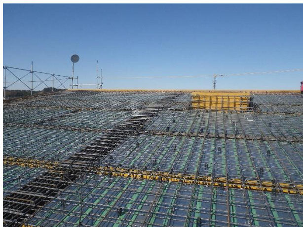
③ 屋根配筋
